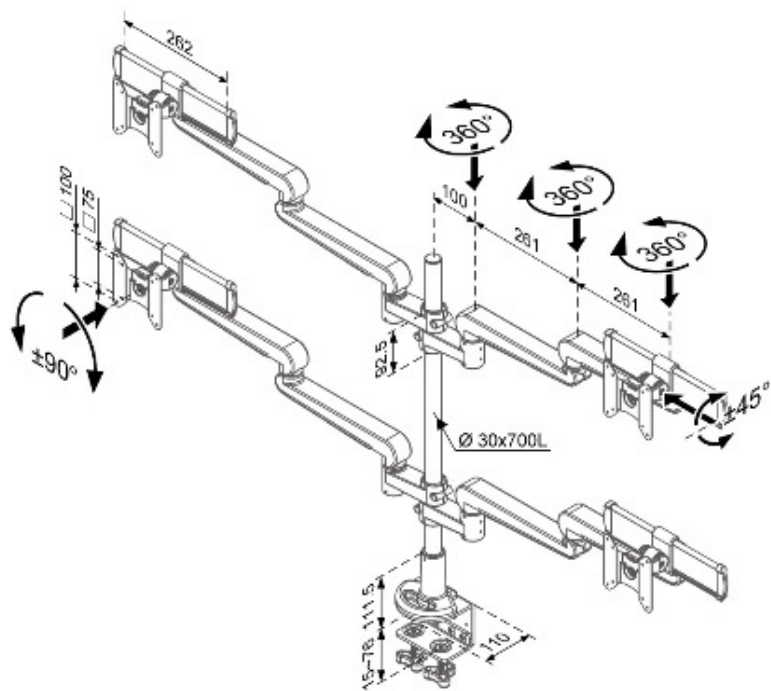
Clamp Type unit:mm
